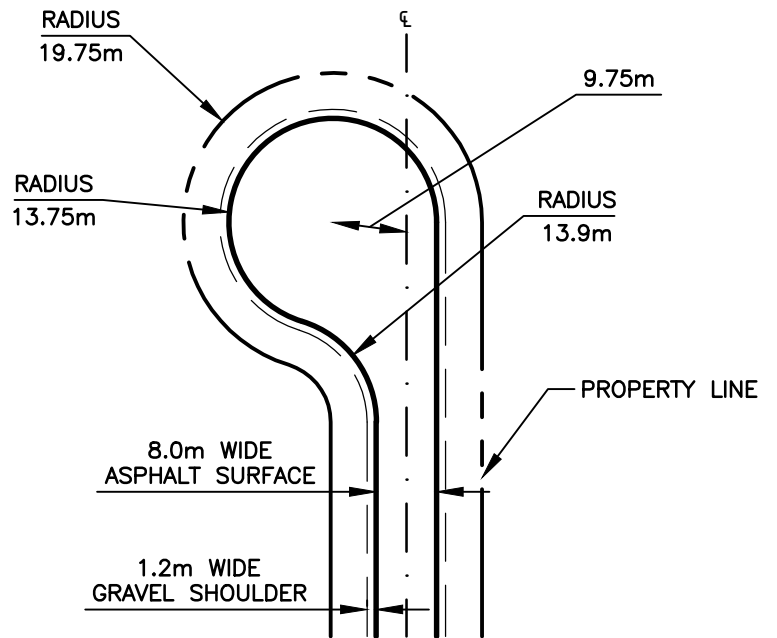
OPTIONAL LAYOUT
